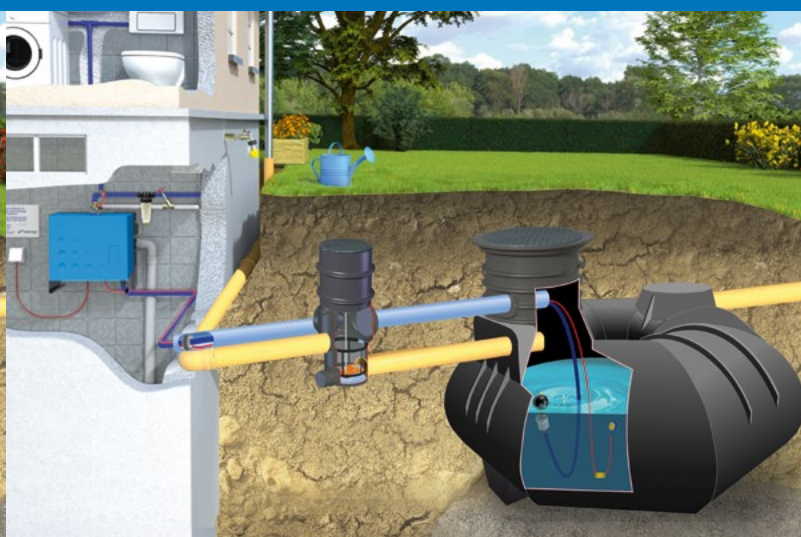
zestaw domowo-ogrodowy OCTAGON standard
