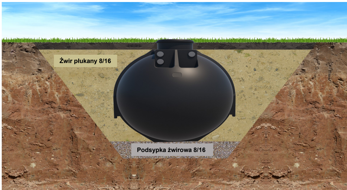
Montaż zbiornika w prostych warunkach gruntowo-wodnych (brak wody gruntowej, grunty przepuszczalne)
