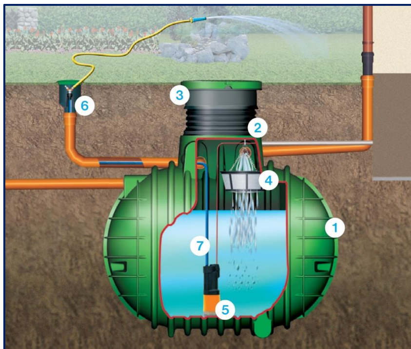
Rys. Schemat instalacji systemu wykorzystania wody deszczowej Garden-Comfort.
